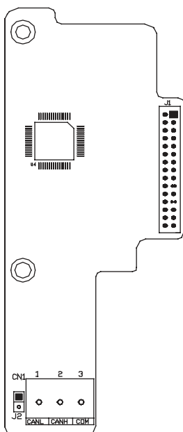
Рис. D-3. Габаритный чертеж платы CANlink
