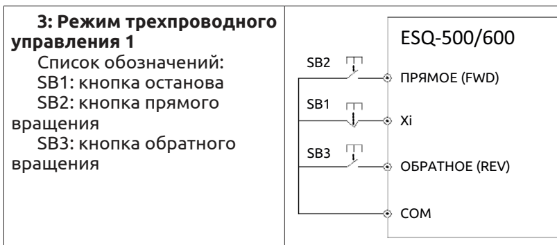
Рис. 7-19 Режим трехпроводного управления 1
