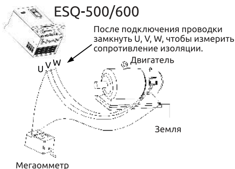
Рис. 1-1 Проверка изоляции двигателя Рис. 1-2 Конденсатор на выходе запрещен
