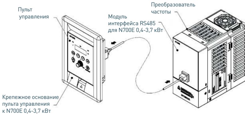
Крепежное основание пульта управления к N700E 0,4-3,7 кВт
