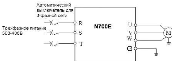
Рисунок 1. Трёхфазная схема подключения мотора к ЧП
