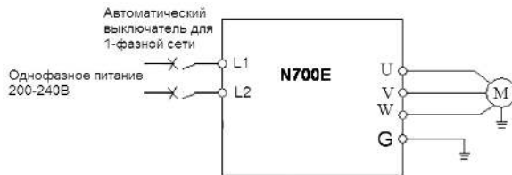
Рисунок 2. Однофазная схема подключения мотора к ЧП
